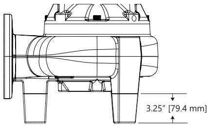
Figura 1. Punto de corte para bombas de 3 a 5 hp
