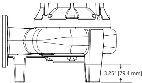
Figura 2. Punto de corte para bombas de 7,5 a 10 hp
